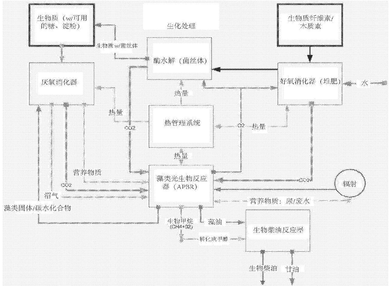
图13生化处理
