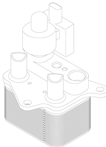
设计1立体图
