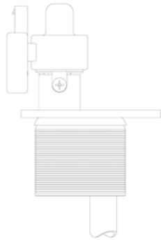
设计2左视图
